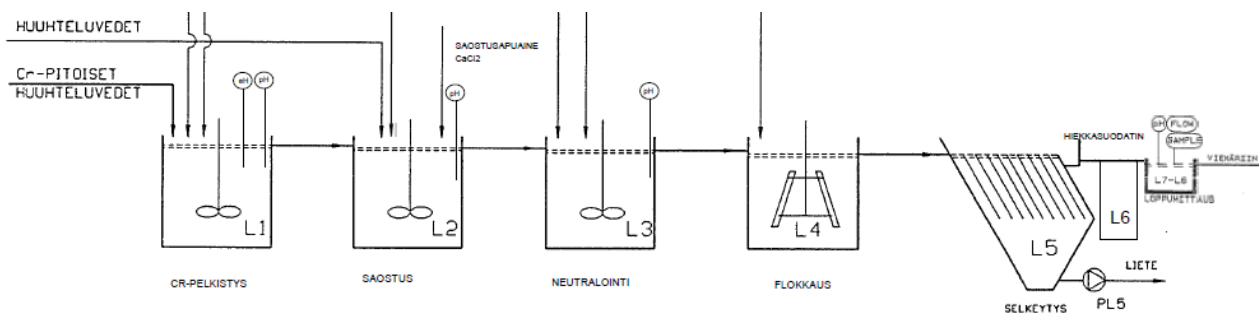
Kuva 9. Prosessikaavio raskasmetallien neutralointilinjasta.
