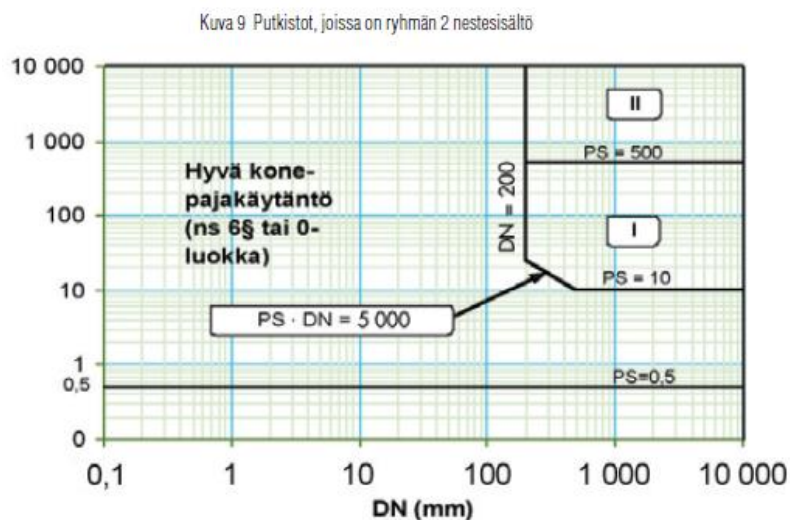
Kuva 8. Ryhmän 2. Putkistoluokitus. /5/
