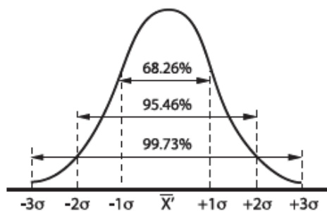
Kuva 4. Normaalijakauma
