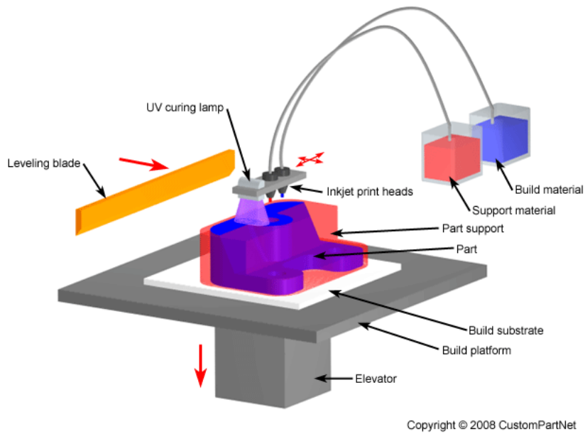
Kuva 2. Materiaalin ruiskutuksen toimintaperiaate (CustomPartNet 2015)
