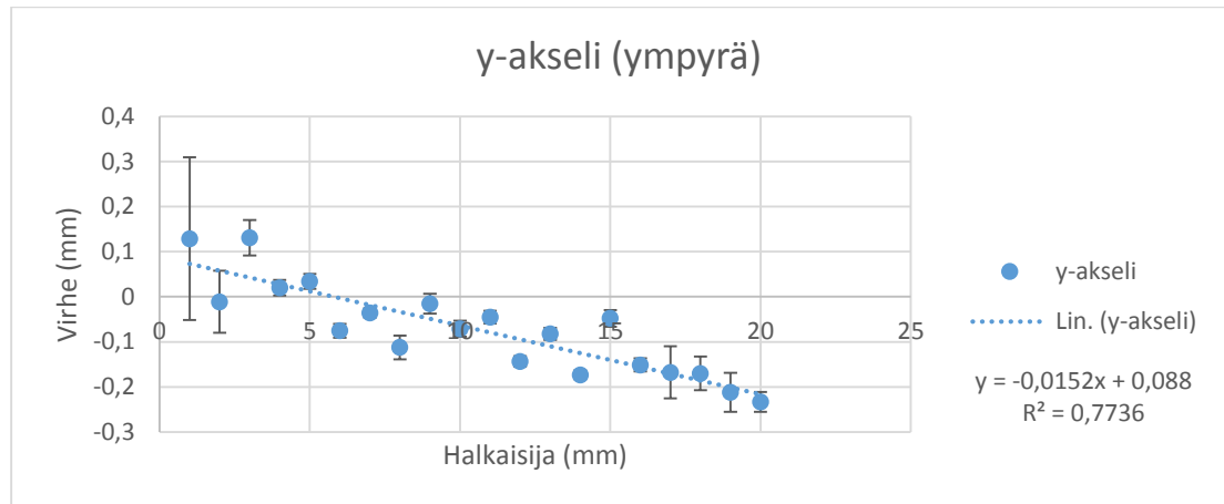
Kuvio 6. Pursotettujen ympyrä kappaleiden y-akselin virheet.
