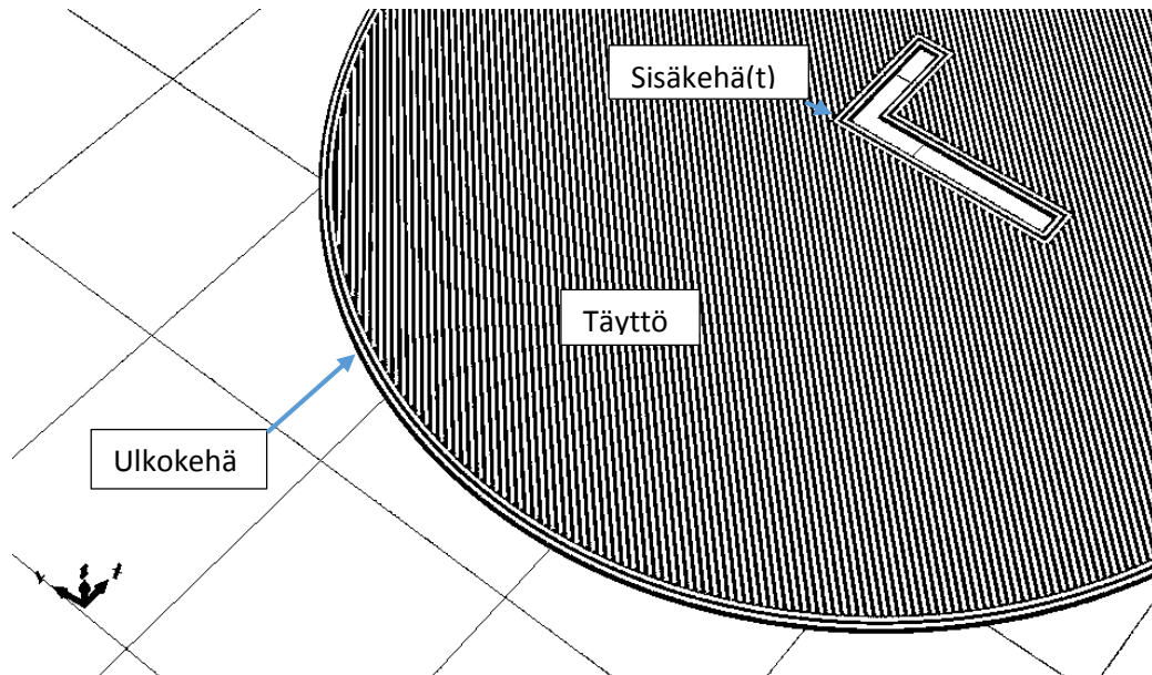
Kuva 16. Esimerkki työstöradoista.
