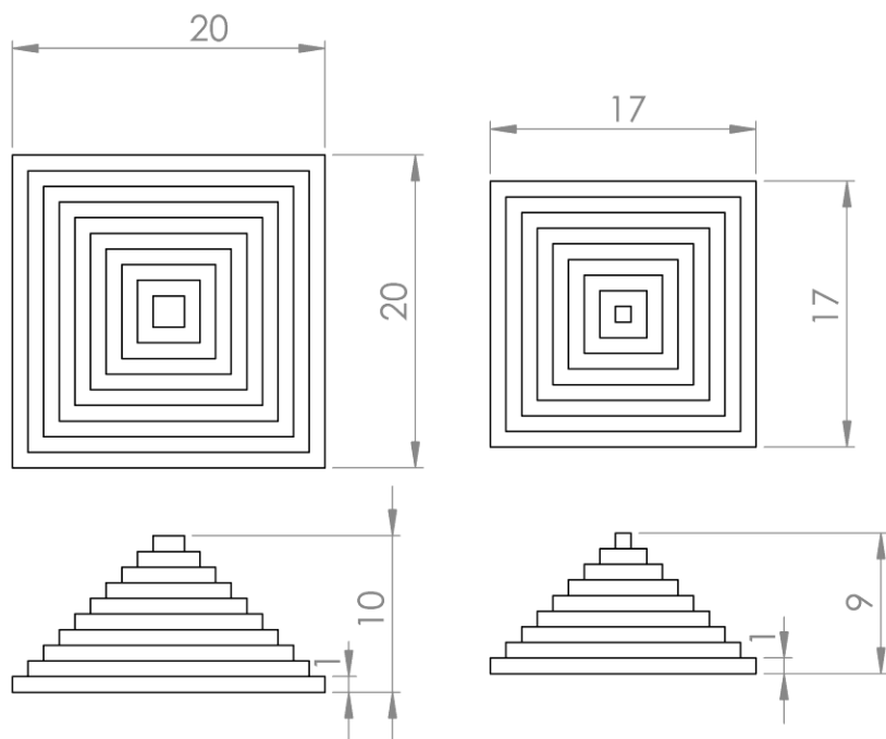
Kuva 19. Mallikappaleiden 4 ja 5 piirustukset
