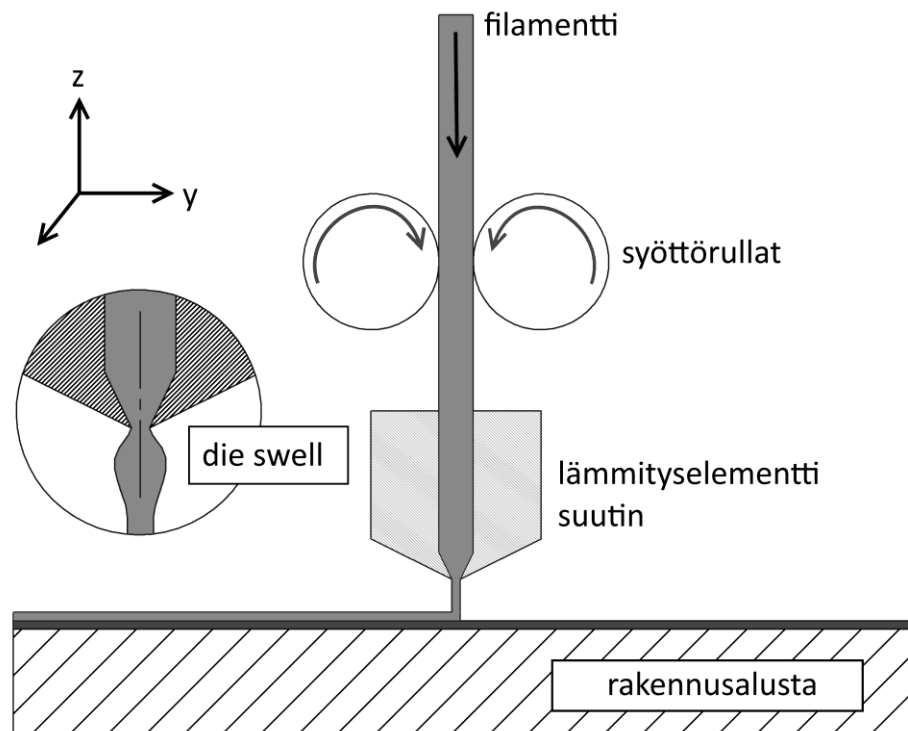
Kuva 15. FFF-menetelmän toimintaperiaate
